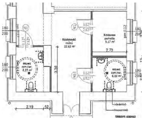
Az északnyugati szárny évtizedekig befalazott földszinti (alagsor) folyosó végi bejáratának tervrajza
